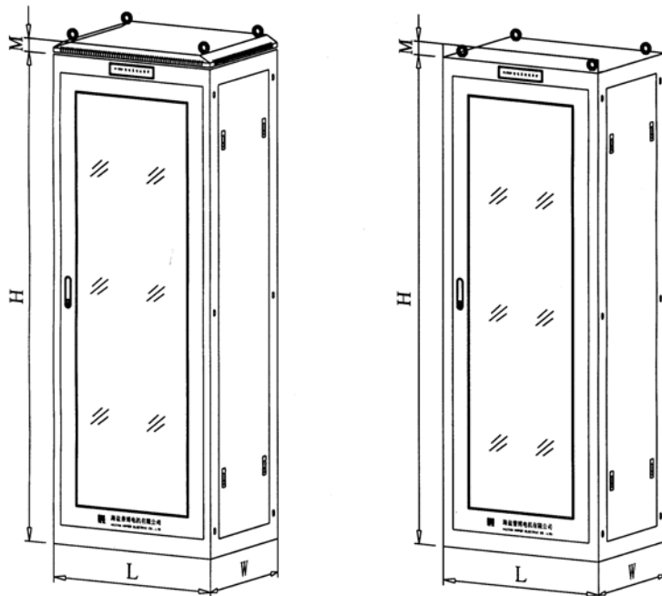
样式一: 顶罩式
